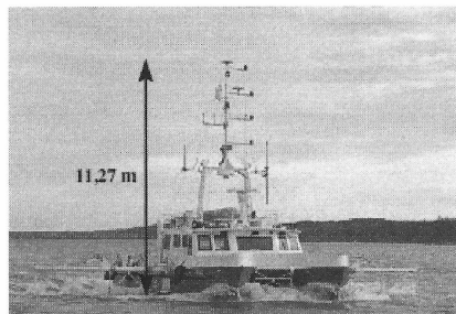
Figure 4 : Navire GC03 utilisé lors des sondages (la différence de hauteur entre l'antenne GPS et la ligne de flottaison du bateau est de 11,27 m). Photographie: courtoisie de la Garde côtière canadienne-Région des Laurentides.
